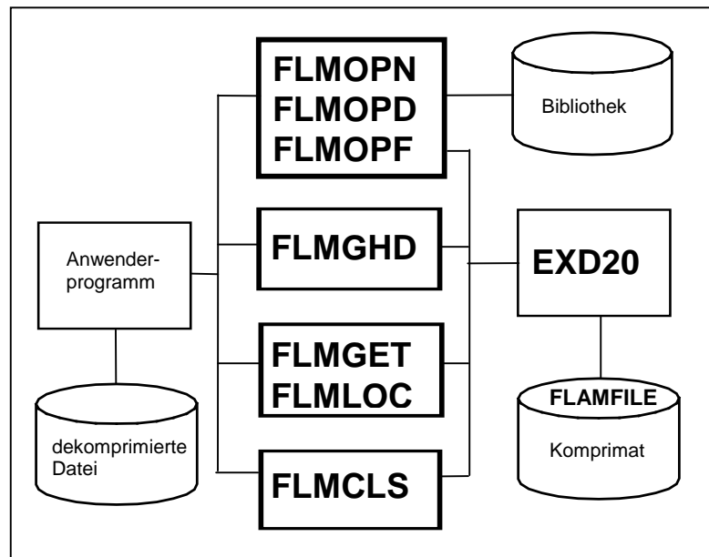
Datenfluss bei Dekomprimierung mit Benutzerzugang
